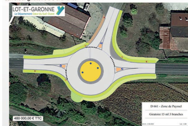
Carrefour giratoire à 3 branches
